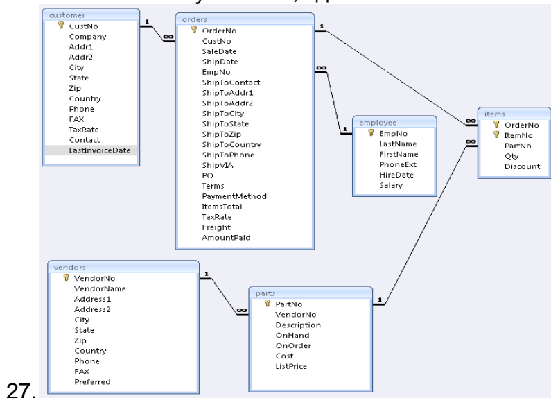
Рис.16. Связь таблиц в демонстрационной базе данных
