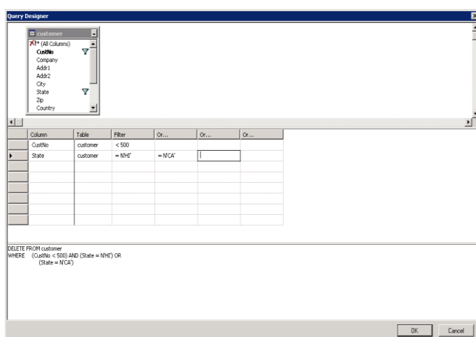
Рис.14. Средства формирования запроса удаления данных
