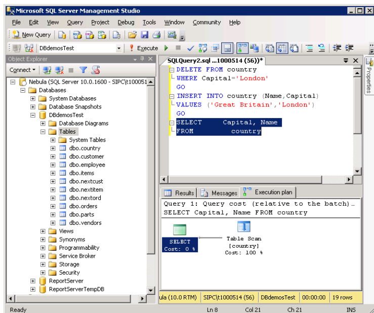
Рис.6. Графическое отображение плана выполнения запроса в редакторе запросов
