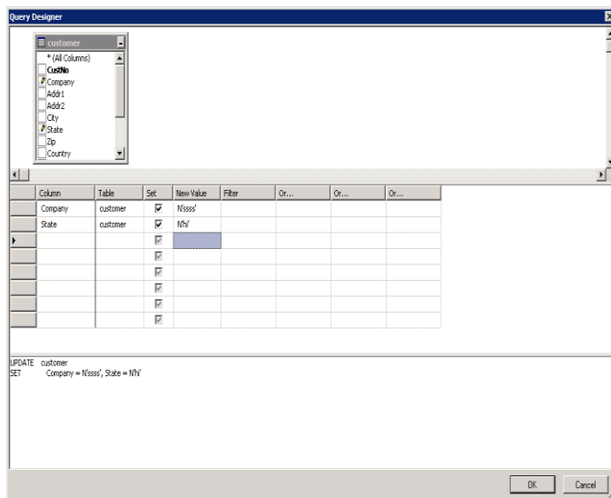
Рис.12. Средства формирования запроса обновления данных
