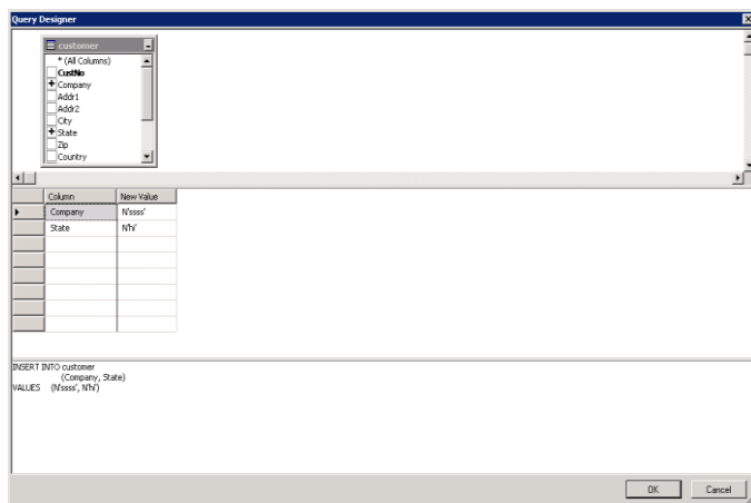
Рис.13. Средства формирования запроса добавления данных
