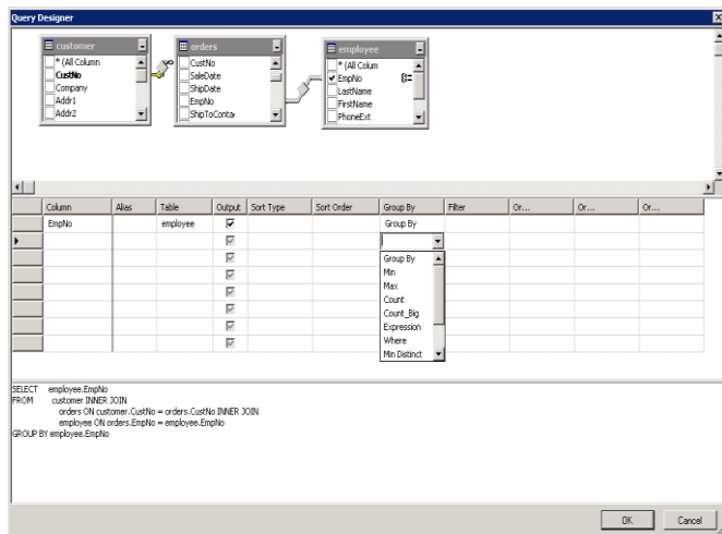
Рис.11. Средства формирования запроса с группировкой
