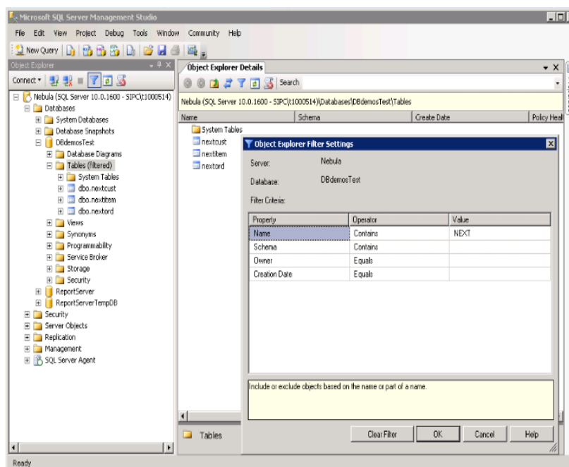
Рис.4. Диалоговое окно Filter Settings (Настройка фильтра) используется для ограничения числа объектов, отображаемых на панели Обзорателя объектов
