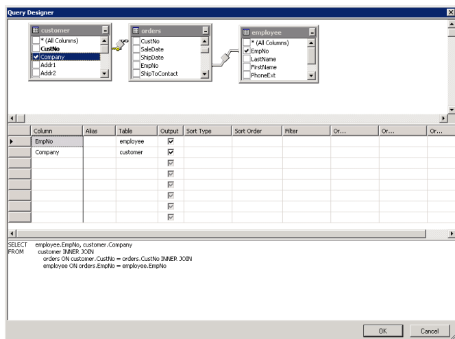
Рис.10. Связь таблиц в многотабличном запросе
